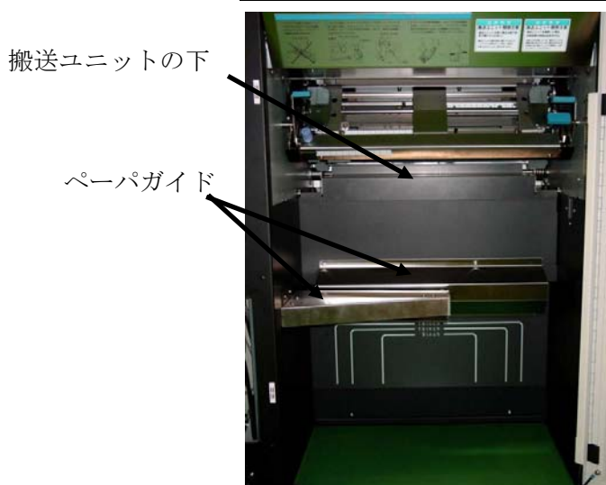
搬送ユニットを開いた状態
