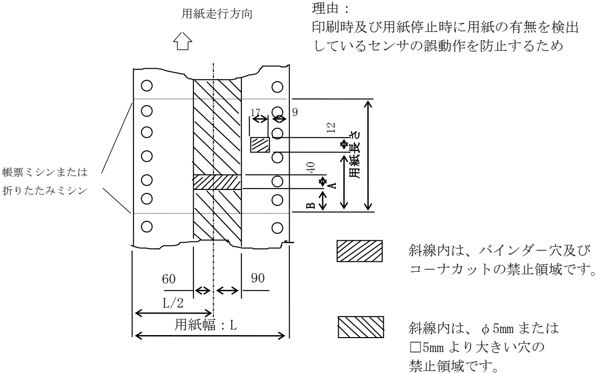
図 B-6 穴あけ禁止領域
